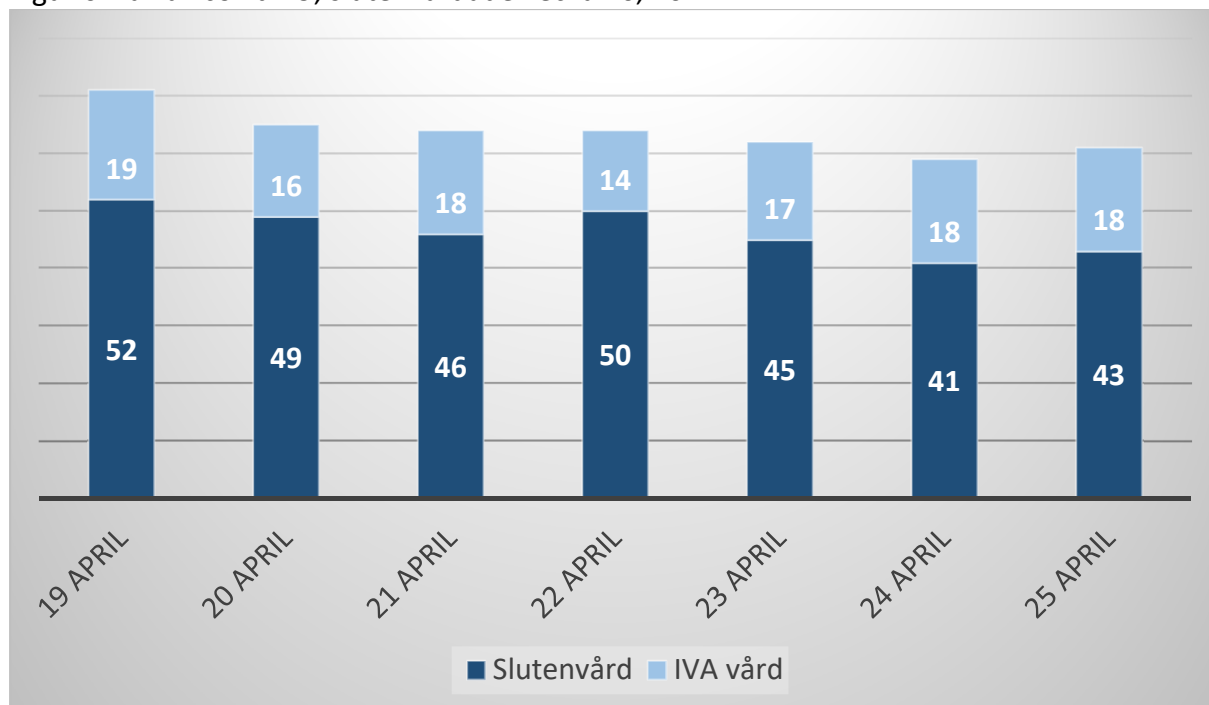
Figur 6. Fall av covid-19, slutenvårdade vecka 16, 2021
