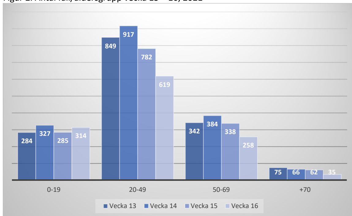
Figur 2. Antal fall/åldersgrupp vecka 13 – 16, 2021
